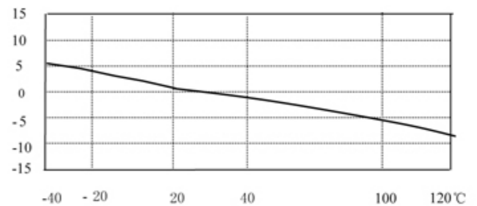
温度曲线
