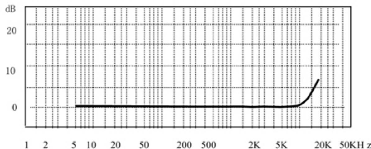
典型频响曲线
