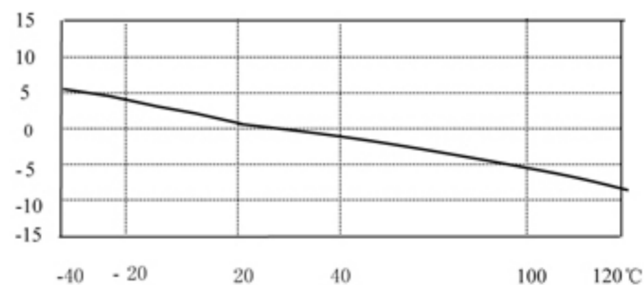
温度曲线
